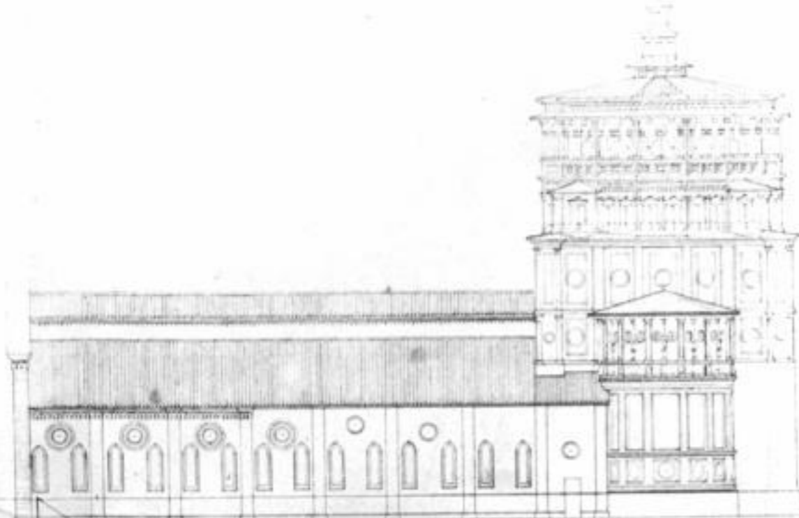
Elevation latérale libre.
